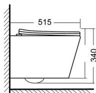
Безободковая конструкция
