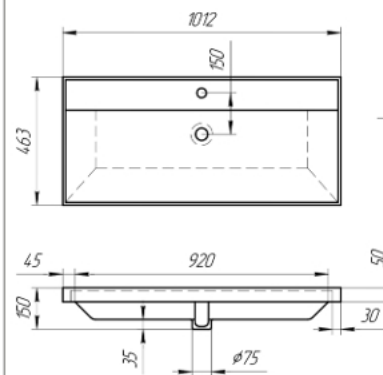
ЭСТЕЛЬ 1000 Мебельный умывальник с переливом
