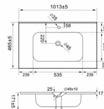
ЭСТЕЛЬ 1000 СЛИМ Мебельный умывальник с переливом
