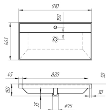
ЭСТЕЛЬ 900 Мебельный умывальник с переливом
