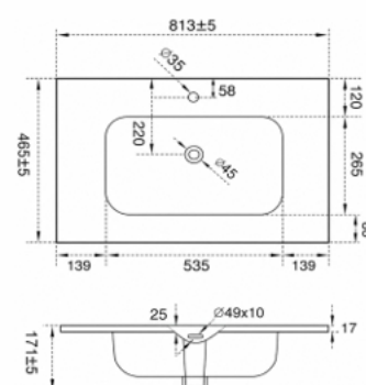
ЭСТЕЛЬ 800 СЛИМ Мебельный умывальник с переливом
