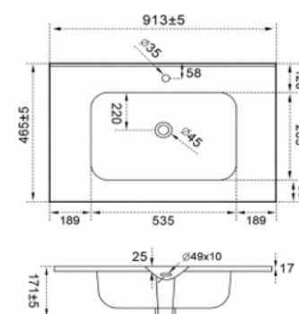
ЭСТЕЛЬ 900 СЛИМ Мебельный умывальник с переливом
