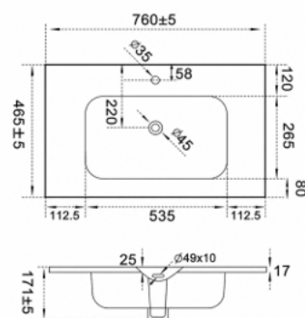
ЭСТЕЛЬ 750 СЛИМ Мебельный умывальник с переливом
