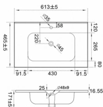
ЭСТЕЛЬ 600 СЛИМ Мебельный умывальник с переливом
